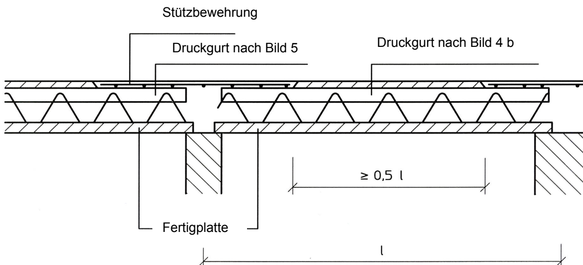
Bild 6: Ausbildung des Betongurtes in Spannrichtung – Mehrfeldplatte
