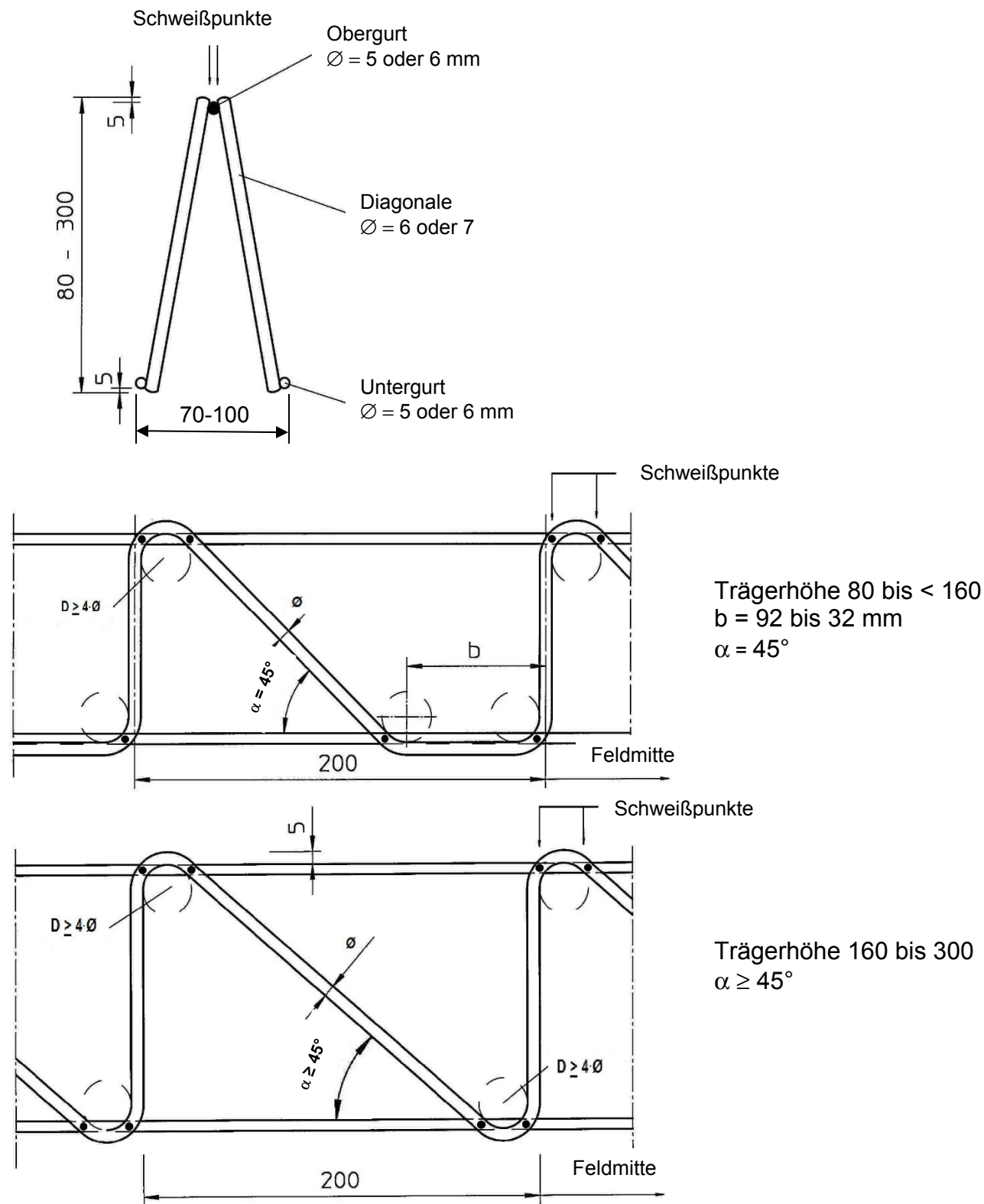
Bild 1: Trägergeometrie
